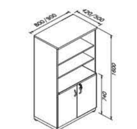
74056 74057 75056 75057 Armário executivo 2 portas baixas
