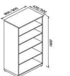
74066SP 74067SP 75066SP 75067SP Armário alto sem portas
