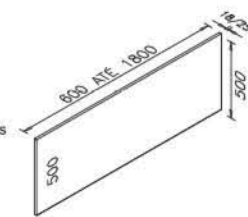
PN75060I PN75080I Mais códigos na tabela de vendas PN75160I PN75180I Painel divisor suspenso inclinado
