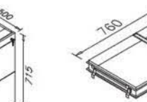
GPS80C GPS80PC Gaveta para pasta suspensa (Armários 800x500)
