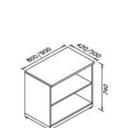
74026SP 74027SP 75026SP 75027SP Armário baixo sem portas
