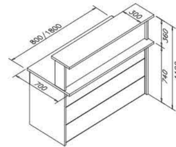
CB75080 CB75100 Mais códigos na tabela de vendas CB75160 CB75180 Complemento retangular para balcão atendimento
